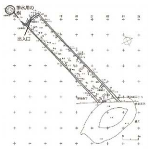
▲アンカリトー9遺跡の掩体壕平面図
